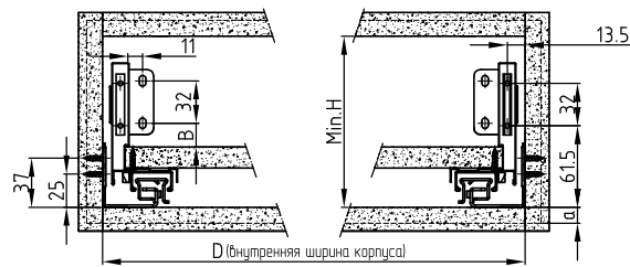
Установочные размеры выдвижного ящика с высотой боковины 80/120 мм
