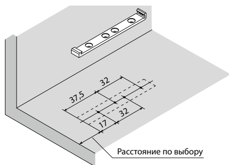
Монтаж ответной части накладного механизма Impulse
