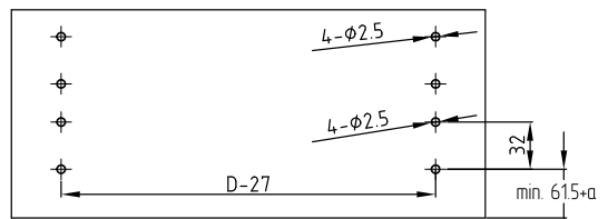
Установочные размеры выдвижного ящика с высотой боковины 80/120 мм и металлическим рейлингом
