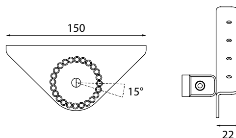
Держатель гардеробной штанги
