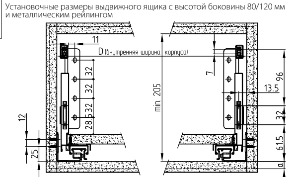
Установочные размеры выдвижного ящика с высотой боковины 80/120 мм и металлическим рейлингом
