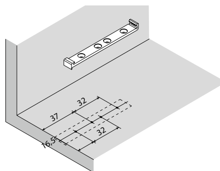
Монтаж ответной части с упором накладного механизма Impulse
